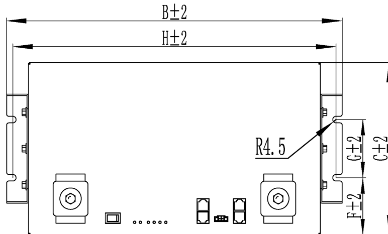
Figure 3-1 Exigences de positionnement d'installation
