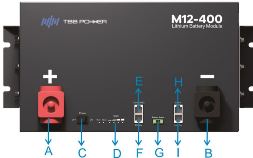
Figure 2-3 Interfaces externes de la batterie lithium M12
