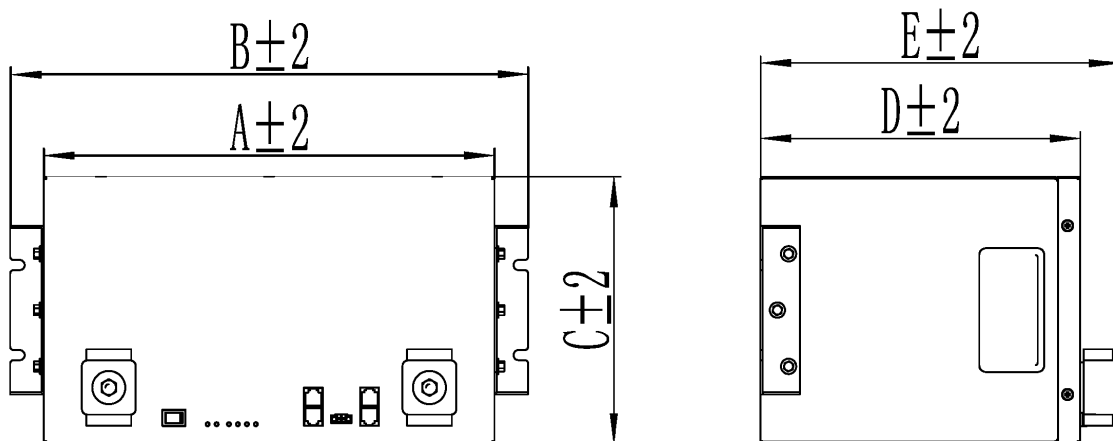
Figure 2-2 Dimensions de la batterie lithium M12
